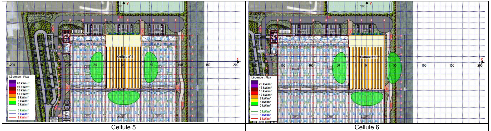
Représentation graphique des distances maximales d'effets thermiques (stockage 1510)
