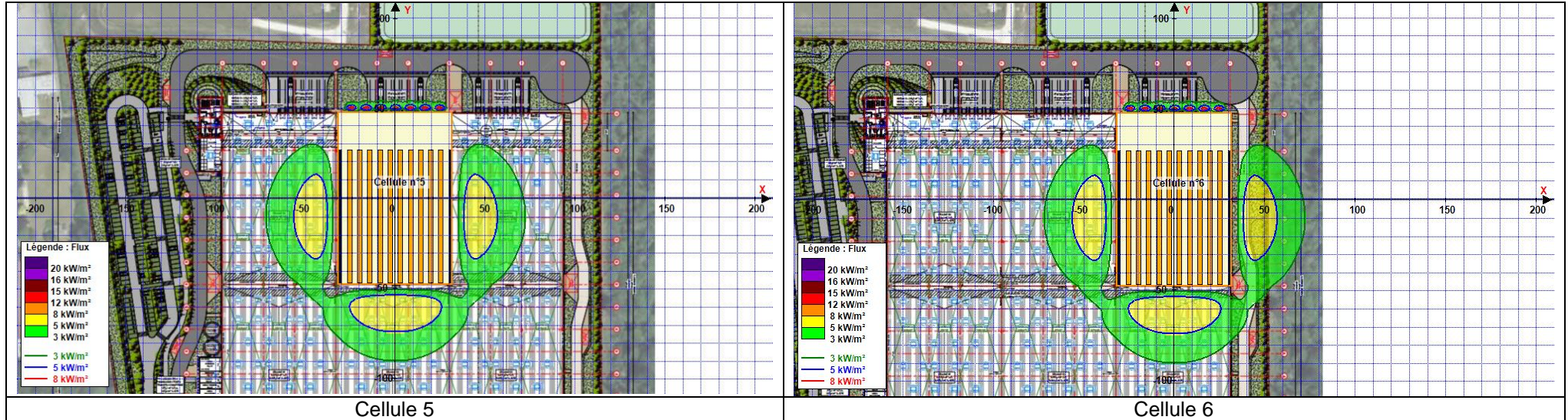
Représentation graphique des distances maximales d'effets thermiques (stockage 2662)
